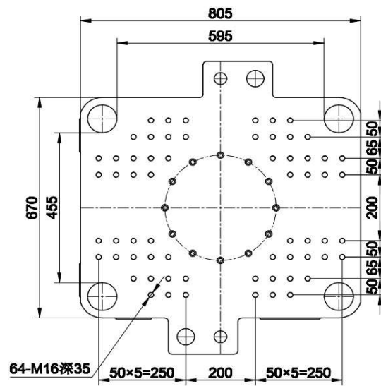
Top Platen
