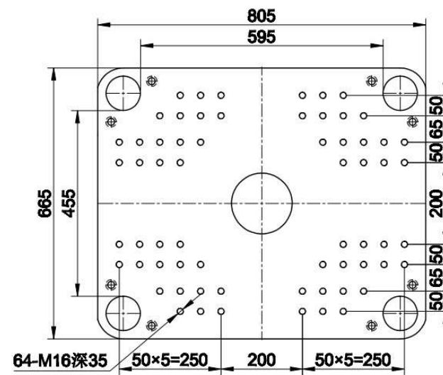
Bottom Platen
