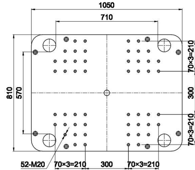
Bottom Platen
