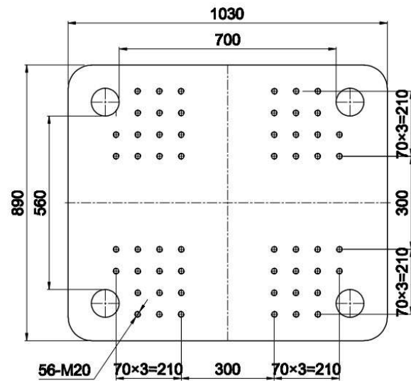
Top Platen
