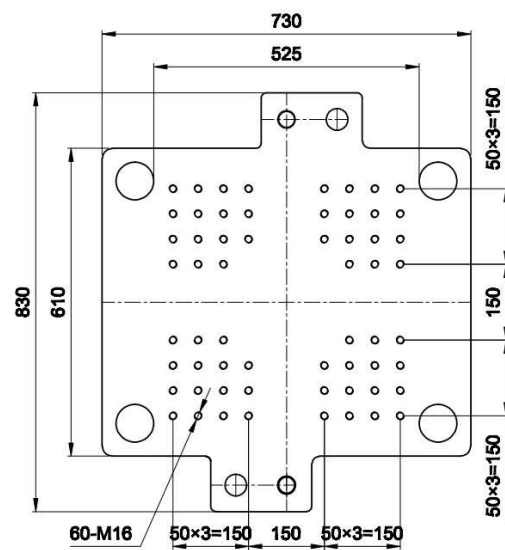
Top Platen
