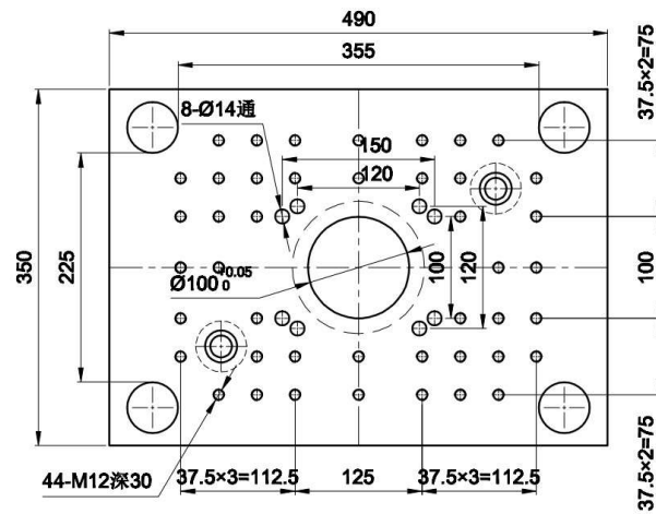
Top Platen
