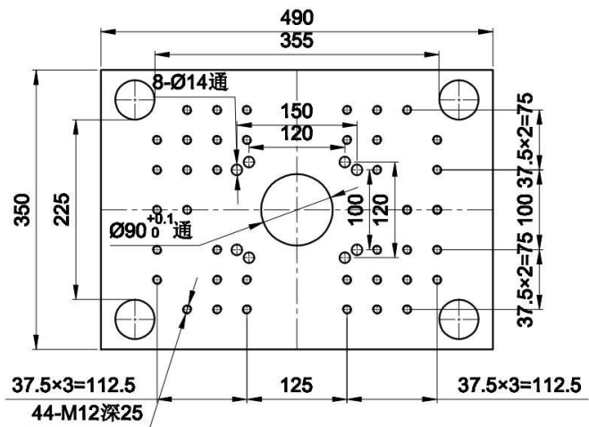
Top Platen
